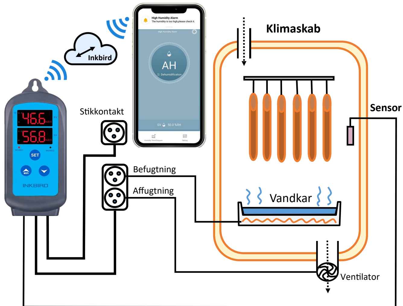
Eksempel på fugtighedskontrol med IHC-200-WIFI
