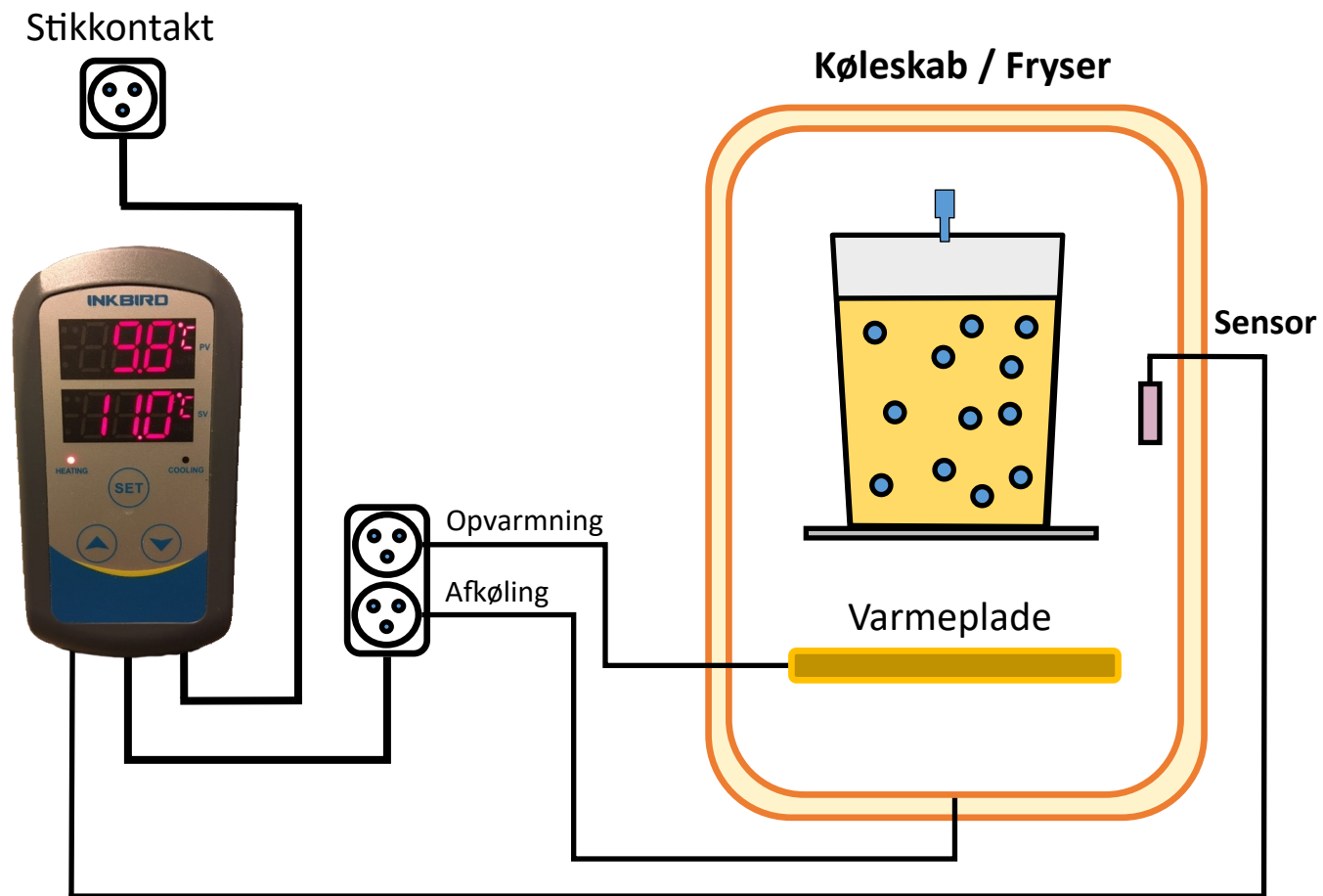
Eksempel på temperaturkontrol med ITC-308, ITC-308 WiFi eller ITC-310TB
